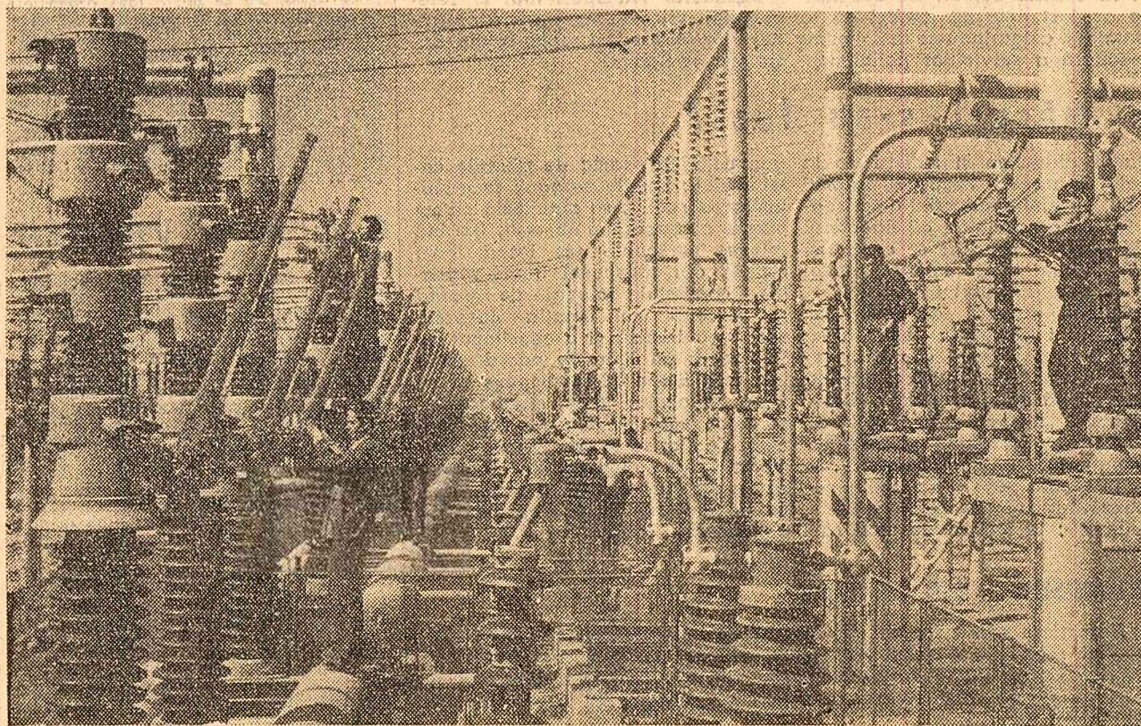
Se montează aparatul de înaltă tensiune la stația de transformare de pe șantierul centralei electrice de termoficare Craiova
