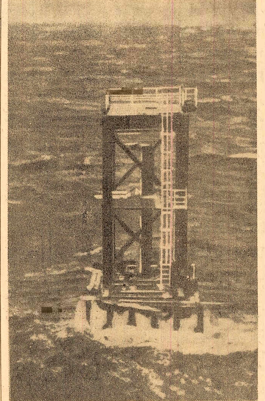
În Marea Nordului a fost amplasată prima bază pentru instalarea unei sonde. Așezată pe patru stâlpi de beton, coborînd la 40 metri adîncime, baza cîntărește 100 de tone și va putea intra în funcțiune. Se prevede extragerea de petrol și gaze naturale
