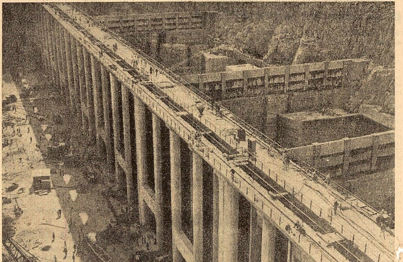
Înainte ca Nilul să-și schimbe cursul; ultimele lucrări la partea subacvatică a clădirii hidrocentralei
