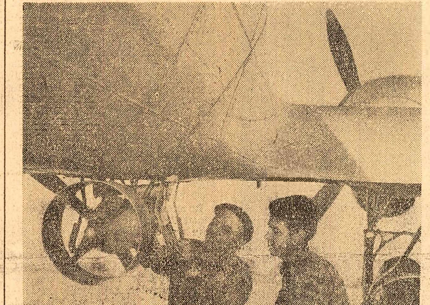
Înainte de zbor se face verificarea sondei cu ajutorul căreia vor fi recepționate variațiile câmpului magnetic al rocilor
