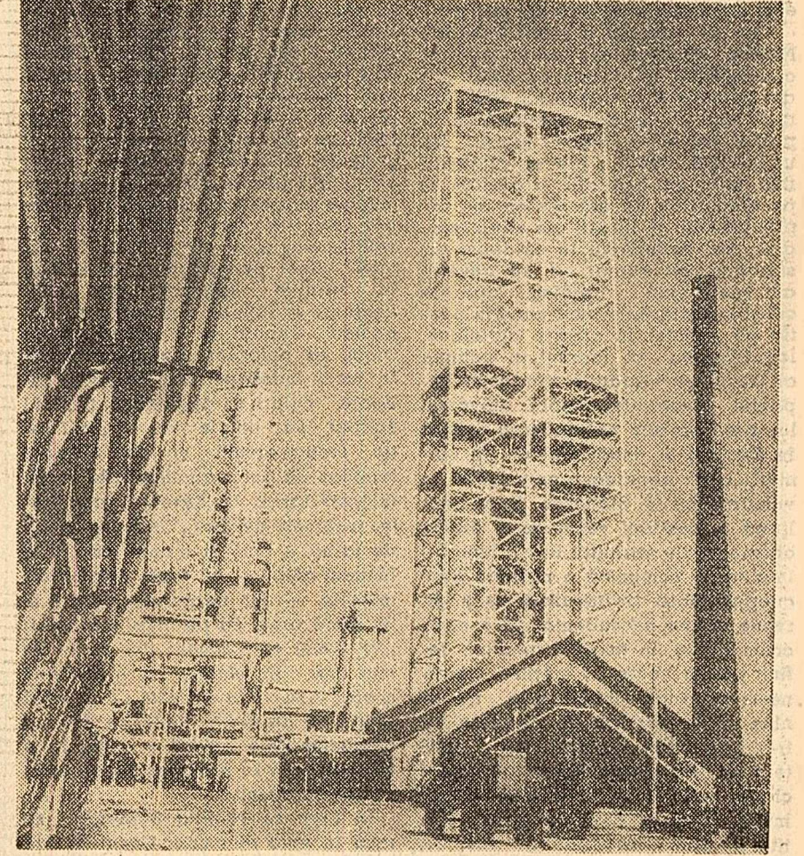
Instalația de cocare întîrziată. Foto Gh. Vințiu
