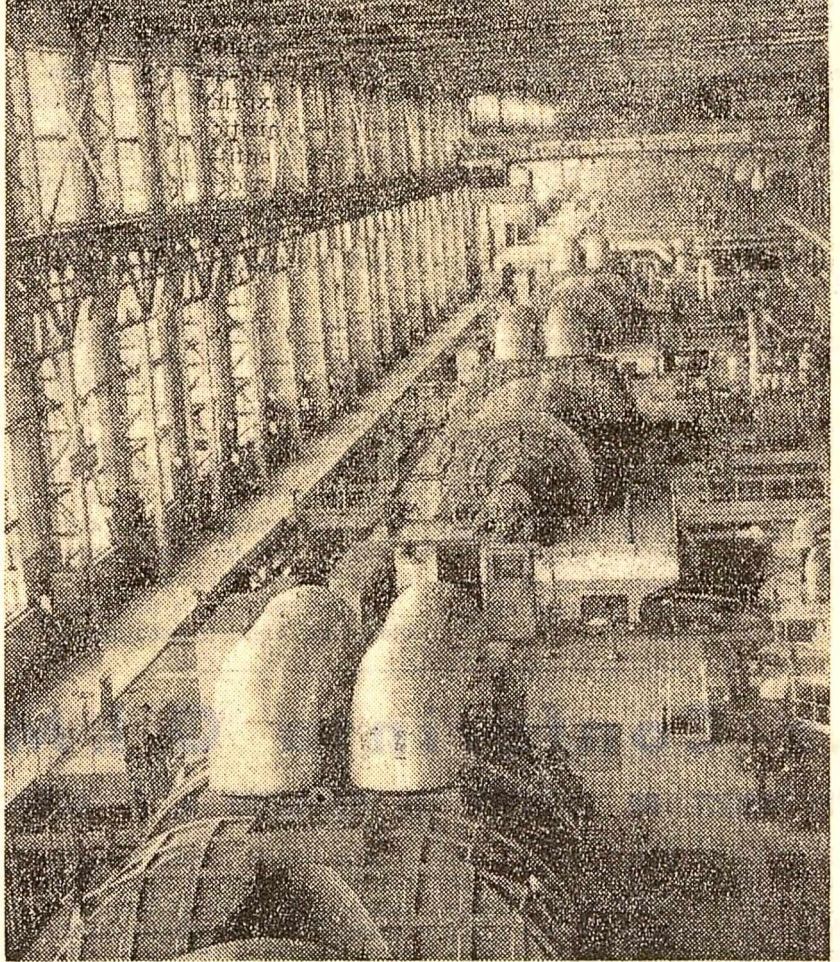
Sala mașinilor centralei electrice „V. I. Lenin” din Staro — Bașevsk (U.R.S.S.). Se montează col de-al nouălea turbogenerator
