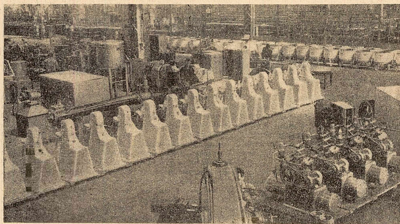
Uzina „Tehnofrig”-Cluj fabrică instalații frigorifice, utilaje și aparatură pentru industria alimentară...
