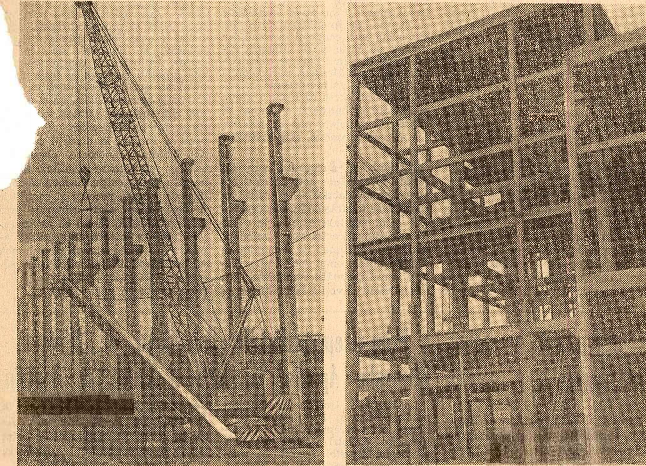
La Combinatul de celuloză și hirtie din Dej. Se montează stîlpii din beton armat prefabricat (stînga). Scheletul halei de regenerare (dreapta)
