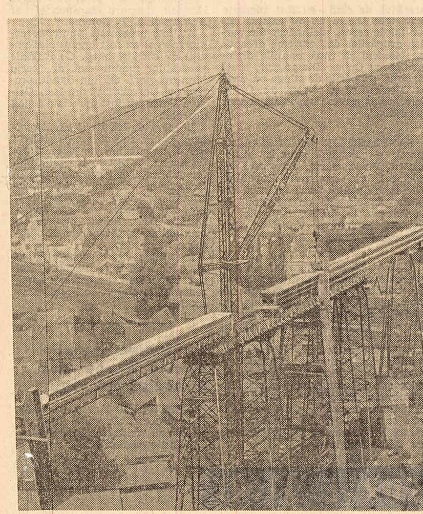
Podul ce se construiește deasupra Reșiței
