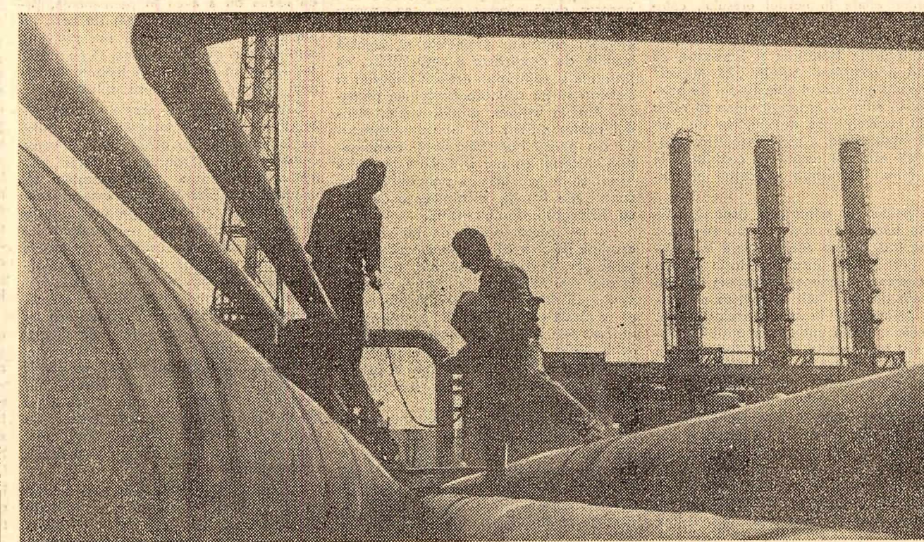
Sudorii la lucru. (Lucrări de montaj pe șantierul Combinatului de îngrășăminte azotoase din Tg. Mureș)
