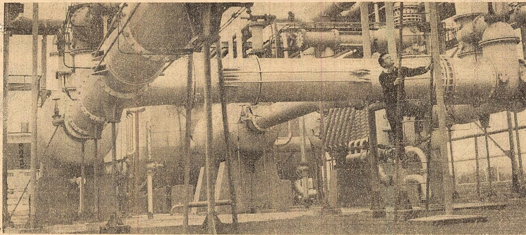
Stația de desbenzinare din școlă Țicleni, regiunea Oltenia
