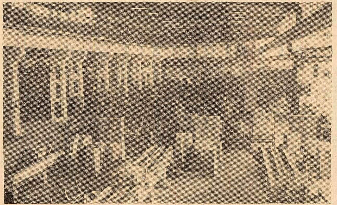
Uzinele Industria Sirmel din Cimpia Turzii. Hala barelor trase. Foto: Agerpres
