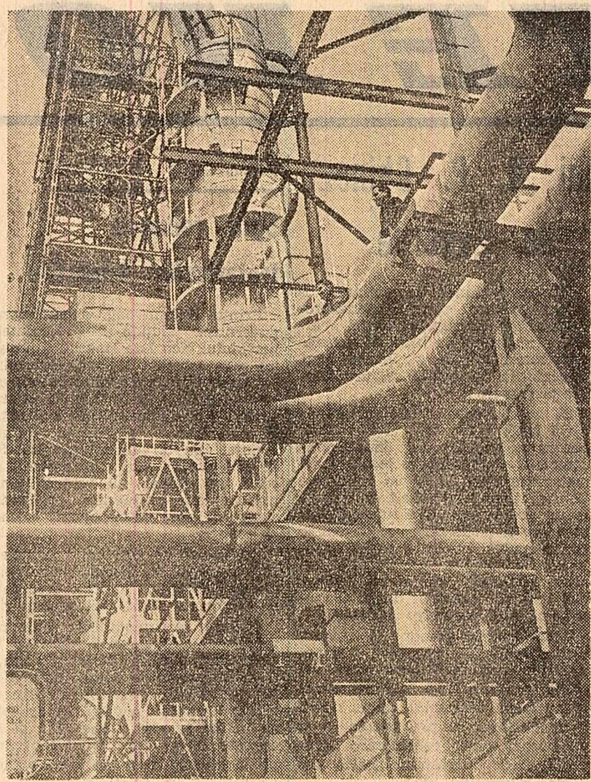
Instalația de cocsare înfiziată de la râlnăria Onești
