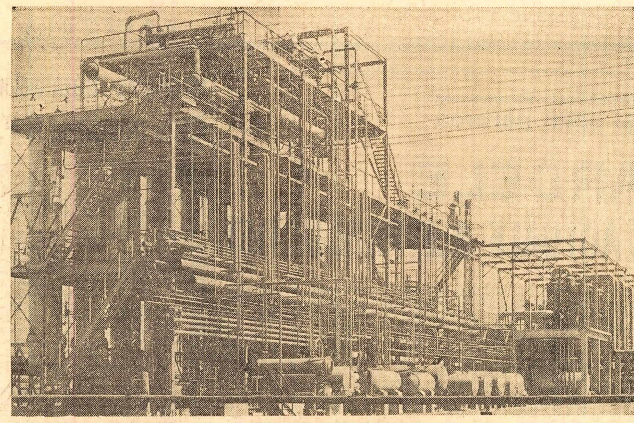
Fabrica de butanoli din cadrul Combinatului pentru chimizarea gazelor naturale din Craiova. Foto: R. Costin
