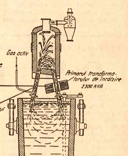
Schema procedurii de degazare prin recirculare
