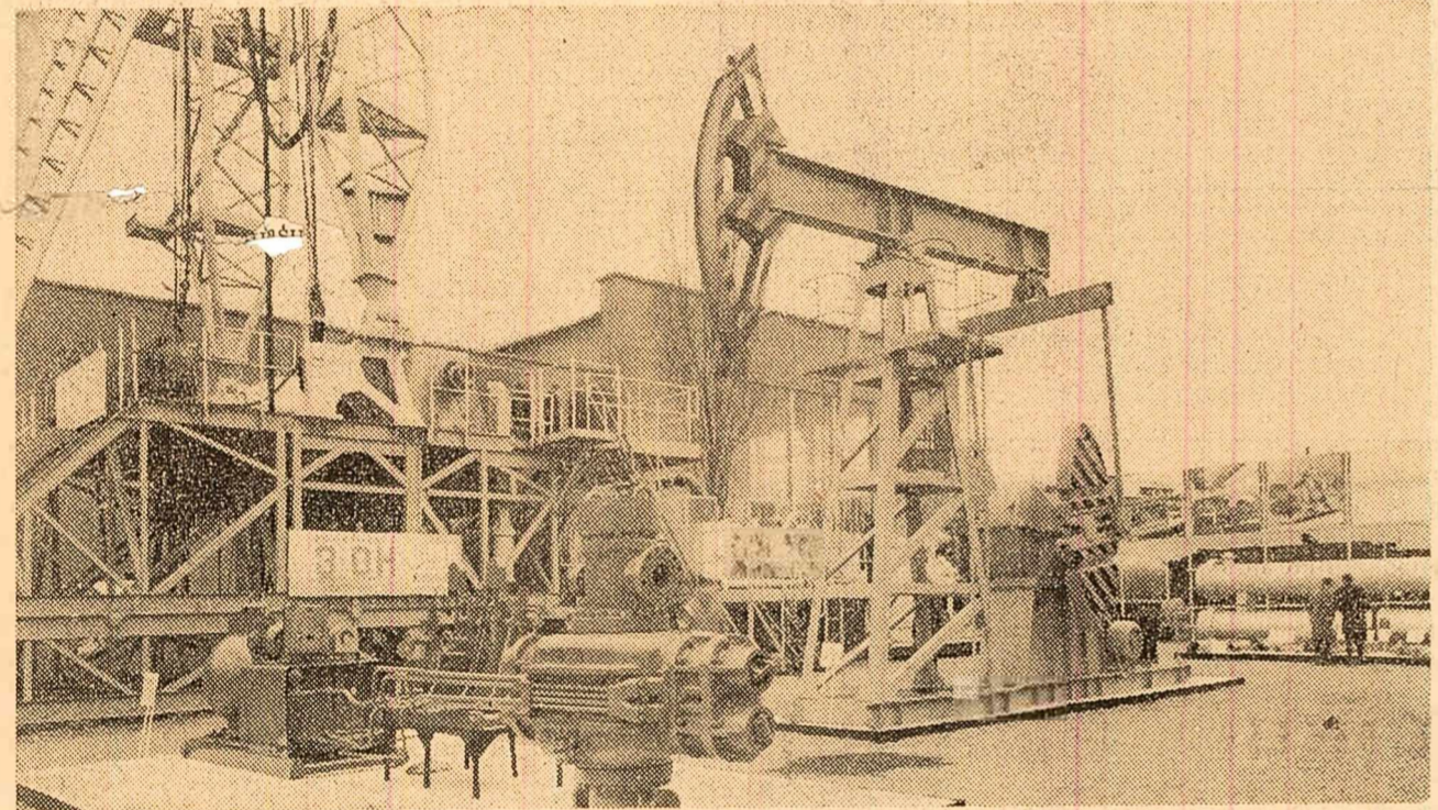
La ediția din primăvara anului 1964 a Tîrgului de la Leipzig, participanții și vizitatorii din diferite țări au manifestat deosebit interes pentru mașinile-unelte de prelucrare a metalelor, locomotiva Diesel-electrică și în mod deosebit pentru instalația de foraj 3 Dh 200.
