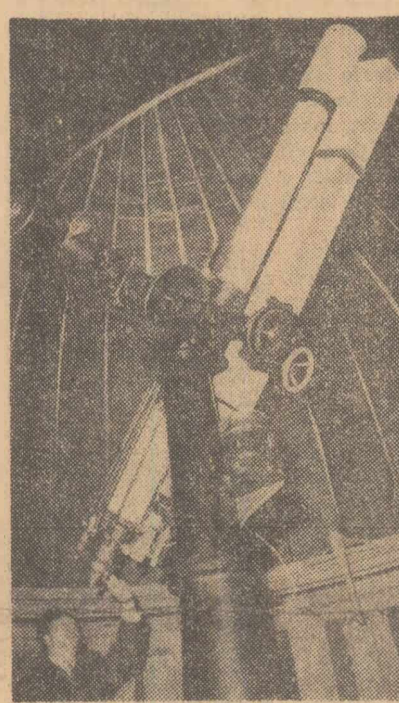
Luneta ecuatorială a Observatorului astronomic popular
