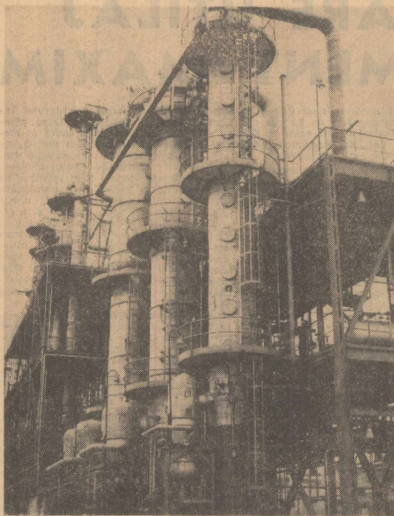
ONEȘTI. Instalația de obținere a stirenului
