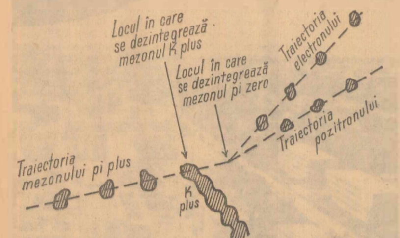
Așa relatează granulele de argint de pe placa fotografică — văzute la microscop — despre dezintegrarea unui mezon K plus și nolle particule care se formează
