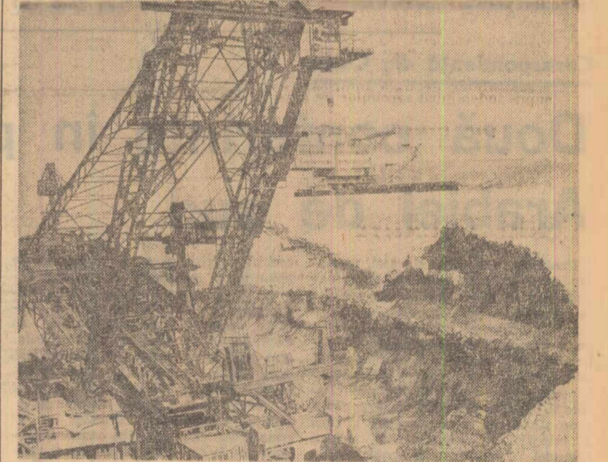
Excavator autopropulsor în funcțiune la exploatarea minieră Turov I, care aprovizionează cu combustibil centrala electrică Turoszow
