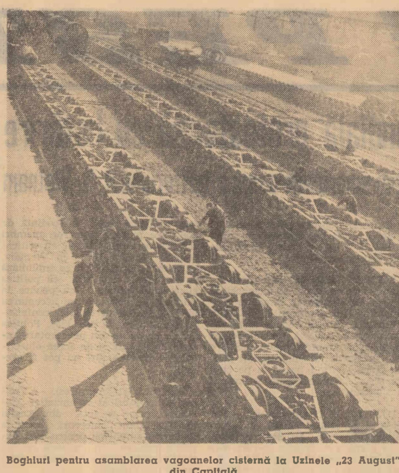
Boghitul pentru asamblarea vagoanelor cisterne la Uzinele „23 August” din Capitală
