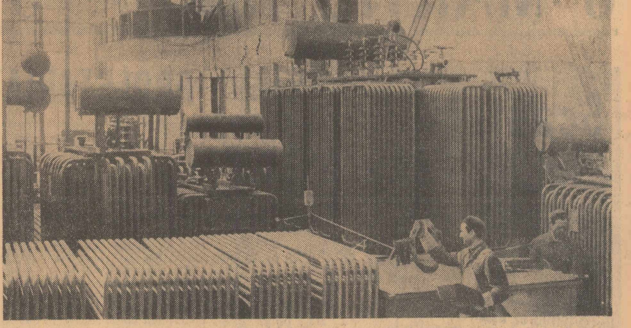
Uzinele „Electroputere”-Craiova: hala de montare a transformatoarelor. Colectivul acestei uzine a primit ieri Steagul roșu și diploma de întreprindere fruntașă pe țară în industria electrotehnică în întrecerea socialistă pe 1964. (În pag. IV-a: relatări de la adunările care au avut loc în diferitele întreprinderi fruntașe, prilejuate de acordarea acestor distincții)
