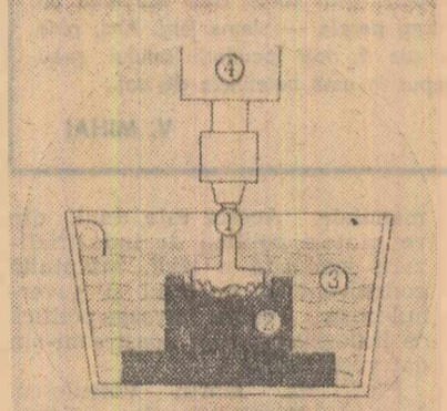
Schema de principiu a prelucrării prin electroeroziune: 1 — electrodul sculă; 2 — piesa de prelucrat; 3 — mediu lichid dielectric; 4 — dispozitiv de reglare
