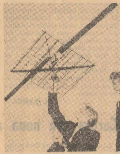
Acest mic „elicopter” realizat în S.U.A. s-a ridicat până la înălțimea de 18 m, fără a avea la bord nici cea mai mică sursă de energie. Forța de propulsie l-a fost furnizată de pe sol prin unde radio
