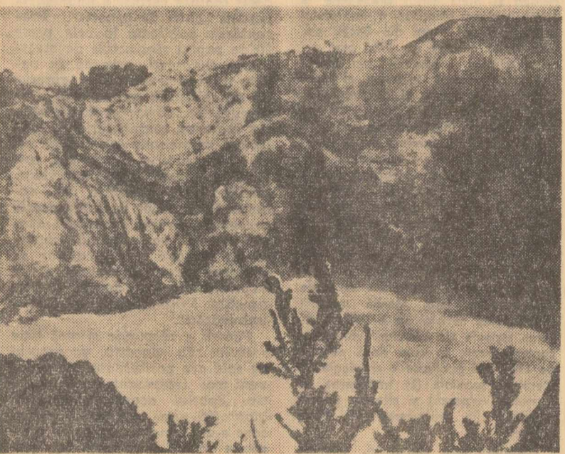
Kawah-Iđjen. Căzind în acest lac vulcanic, format dintr-un amestec de acizi sulfurici și clorhidrici, bucăți mari de roci calcareoase se dizolvă în clocele
