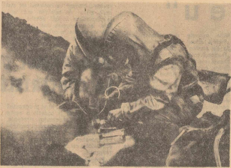
Stromboli. Prima folosire la fața locului a noului aparat pentru analiza gazelor vulcanice
