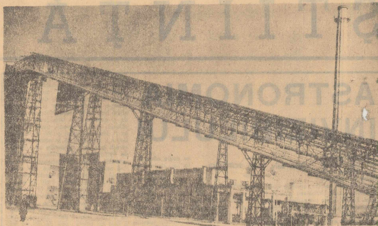
În prima decadă a lunii martie, colectivul Uzinei de produse sodice din Govora a produs peste plan 1114 tone sodă calcinată, 212 tone sodă caustică și 60 tone silicai de sodiu. În fotografie: Instalația de încălzire automată a cuploarelor
