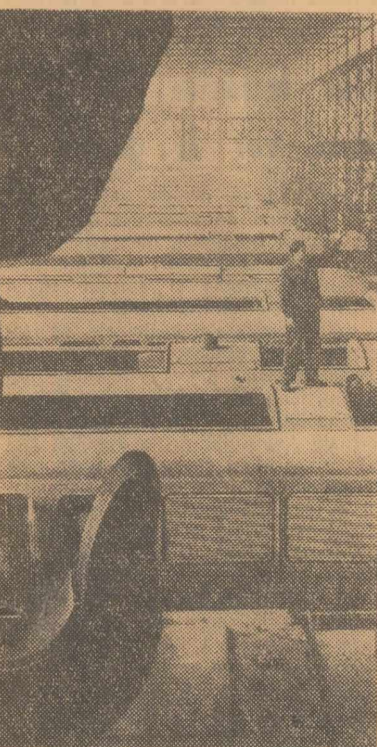
Secția de montaj general a locomotivelor Diesel de la uzina „Electroputer” din Craiova
