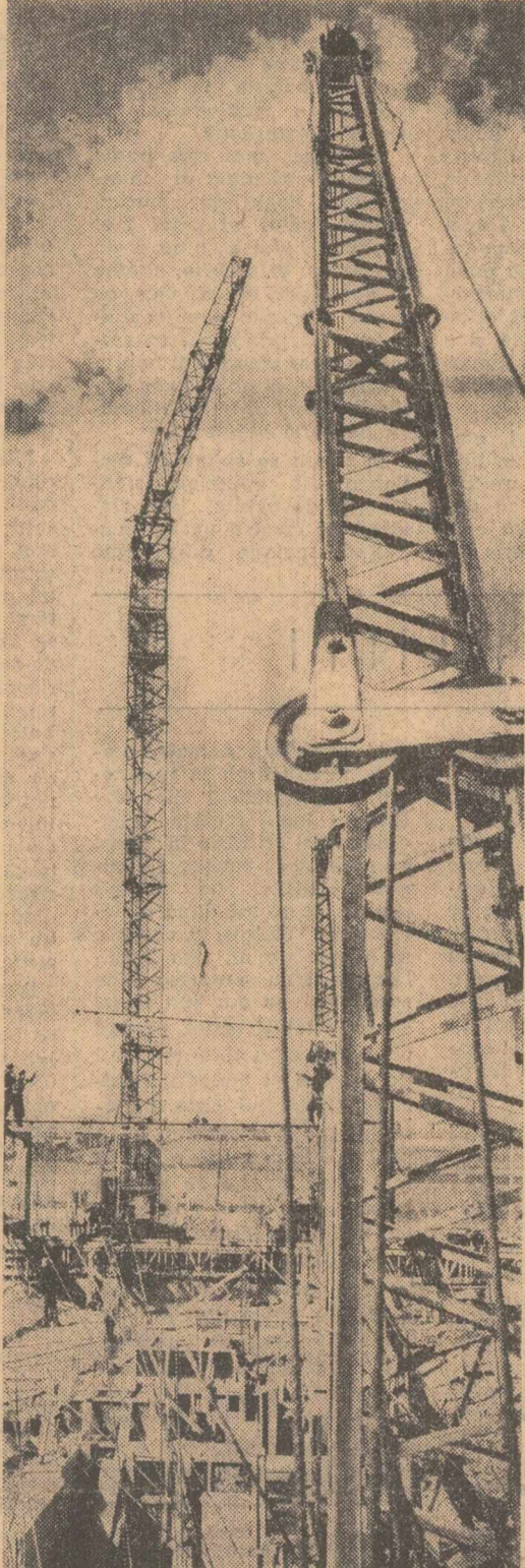
Pe șantierul centralei electrice de termoficare București Sud
