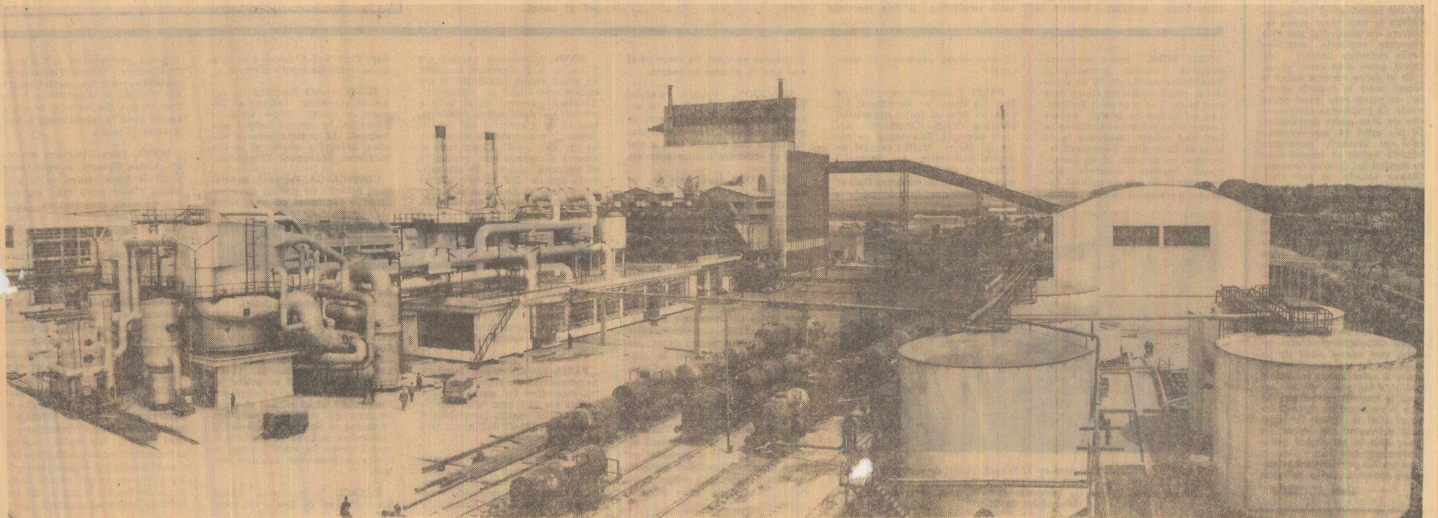
Fabrica de acid sulfuric de la Combinatul de Îngrășăminte chimice Turnu Măgurele
