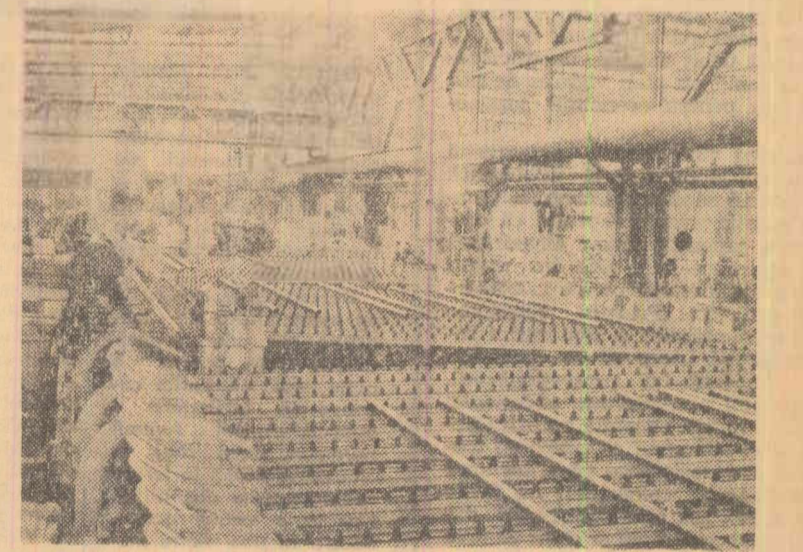
Linia laminorului Stiel de la uzina siderurgică din Kuncice (R. S. Cehoslovacă)
