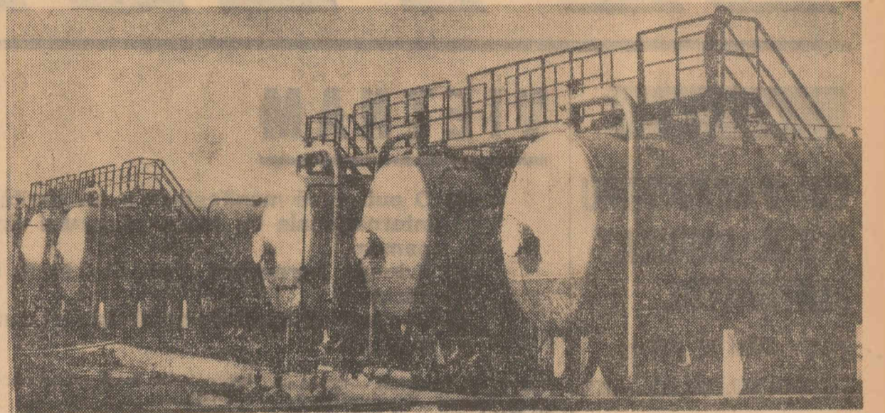
Stația de dezbenzinare de la școala Clujești (Argeș). Vedere parțială a instalației de tratare a fiivelului
