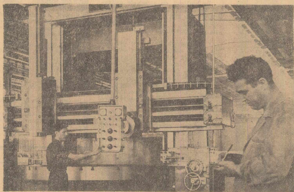
Ultimele probe și un nou strung carusel de 2 500 mm, construit la Fabrica de mașini-unelte și agregate din Capitală, este gata pentru livrare
