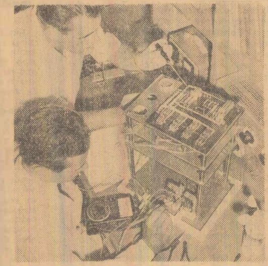
Se verifică subsansamblele stației meteorologice automate. Foto: M. Cluc
