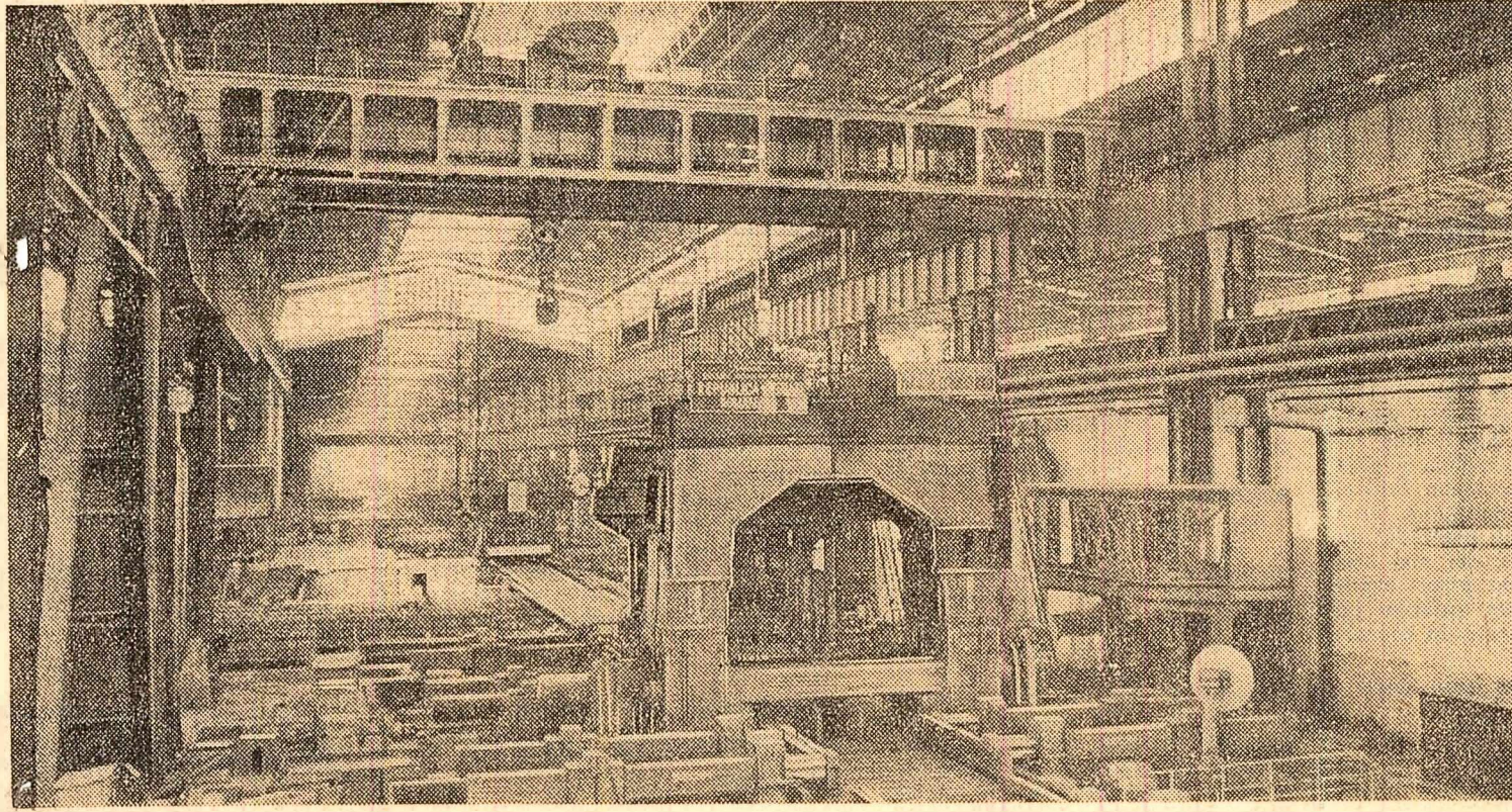
Urtașa „seră” de 110 000 m.p. a laminorului de tablă groasă de la Galați. Se află aici în curs de montare numeroase utilaje tehnologice
