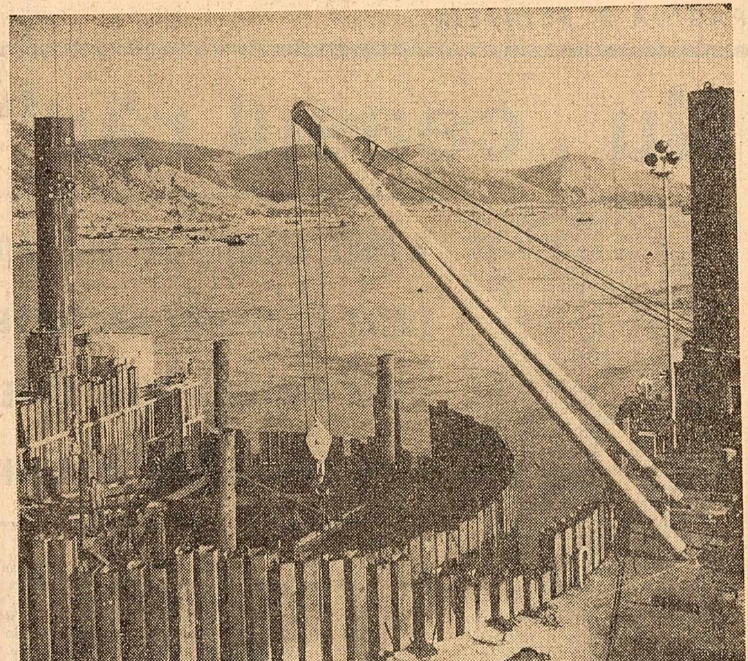
A fost montată prima celulă a bataradoului ce va devia apele Dunării la Porțile de Fier Foto: Gh. Vlădăreț
