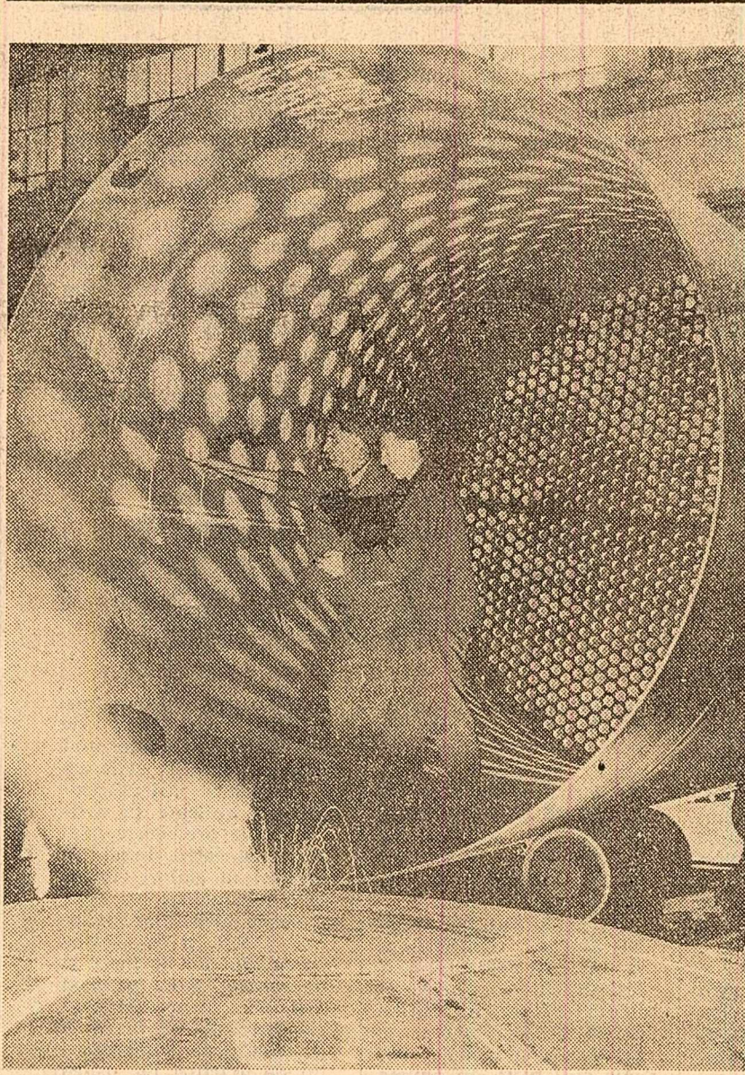
La Uzinele „Vulcan” se trasează interiorul unui reactor pentru Combinatul chimic de la Turnu Măgurele
