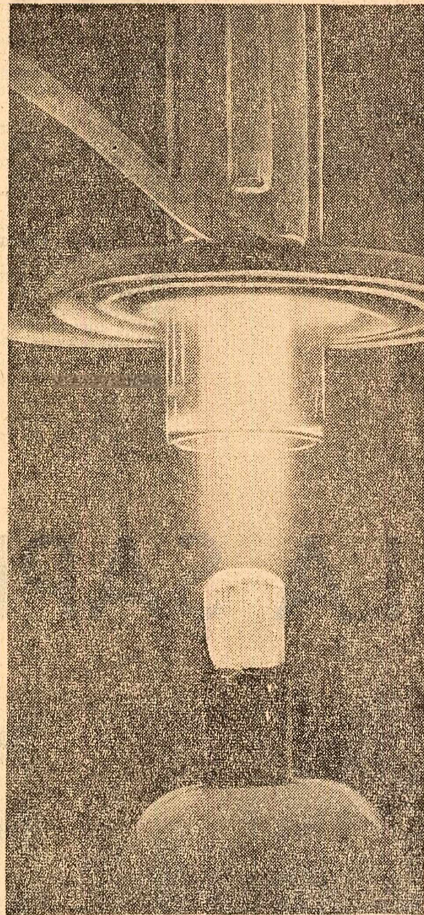
Multe aparate moderne de cercetare, în special în domeniul spectroscopiei, au nevoie de cristale în cantități și de dimensiuni științifice „Mantred von Ardenne”, din R. D. Germană, a fost realizat pentru „creșterea” cristalelor acestor arzător cu plasmă, acționat prin curenți de înaltă frecvență
