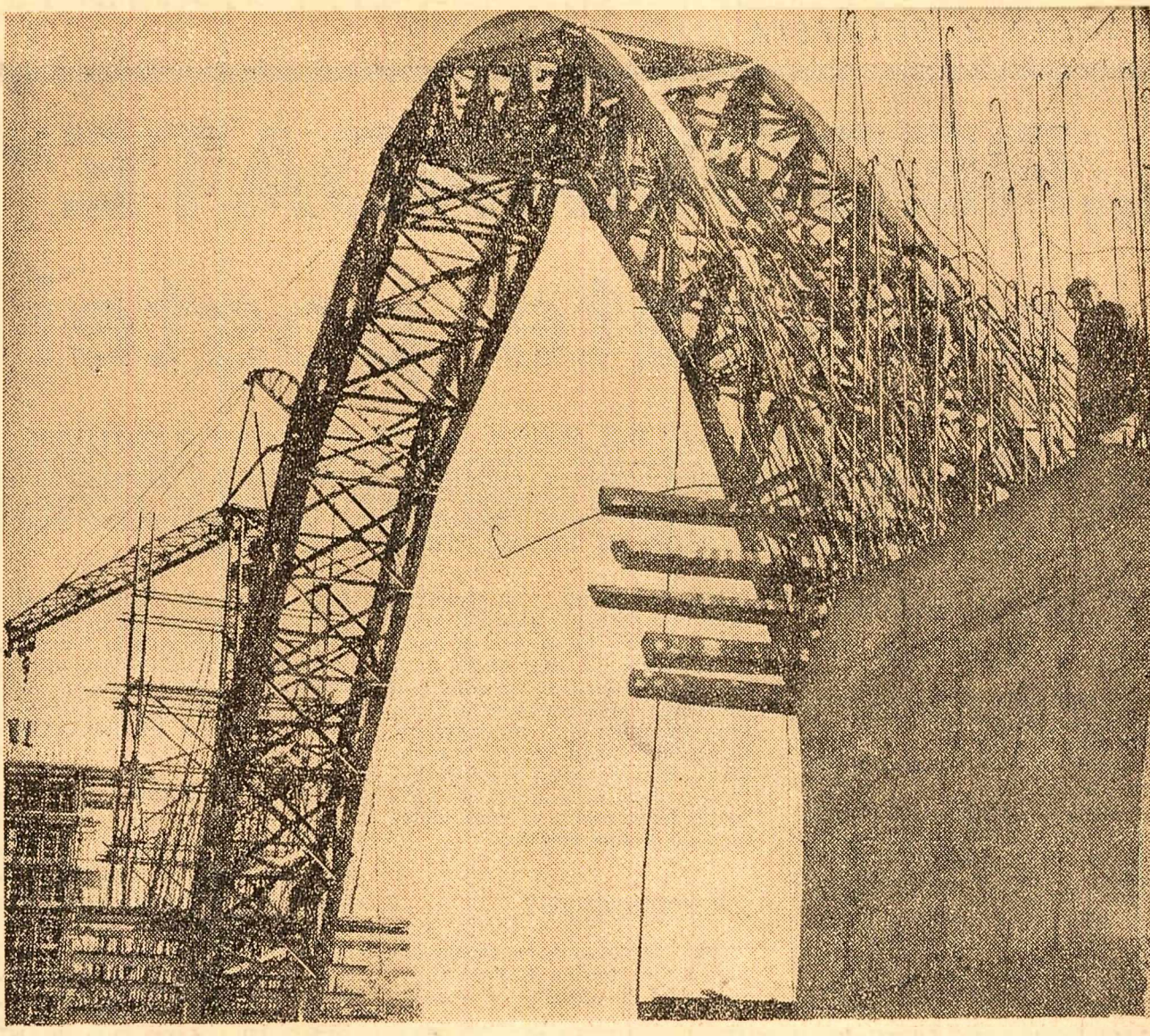
Unul din viaductele în construcție pe noul traseu al liniei de cale ferată de la Porțile de Fier
