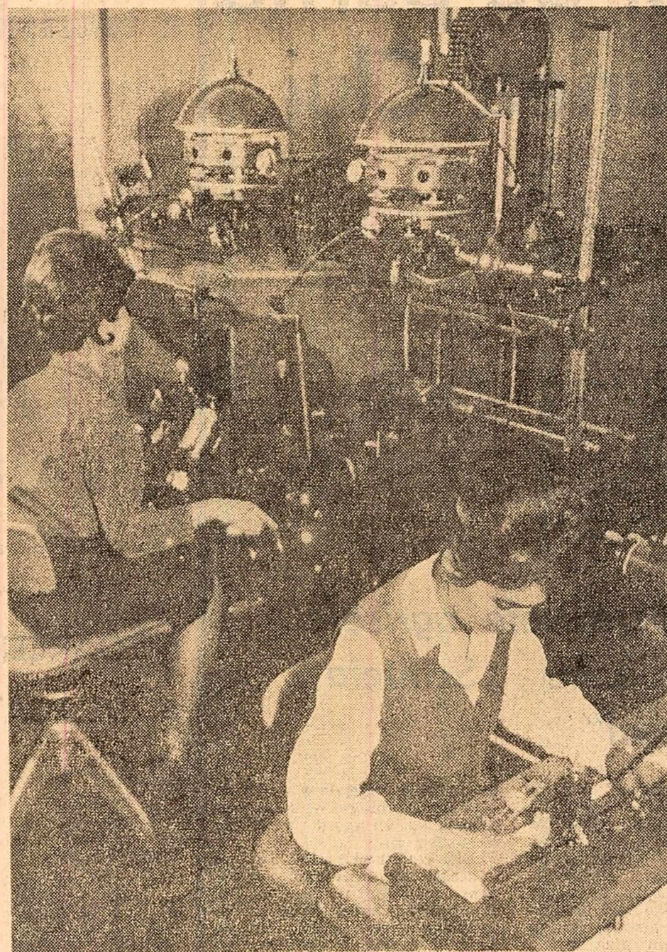
„Autograful” — un aparat optic complex — permite transformarea fotografemelor, luate din avion, prin eliminarea tuturor deformărilor datorate perspectivei sau oscilațiilor, în hărți de mare precizie
