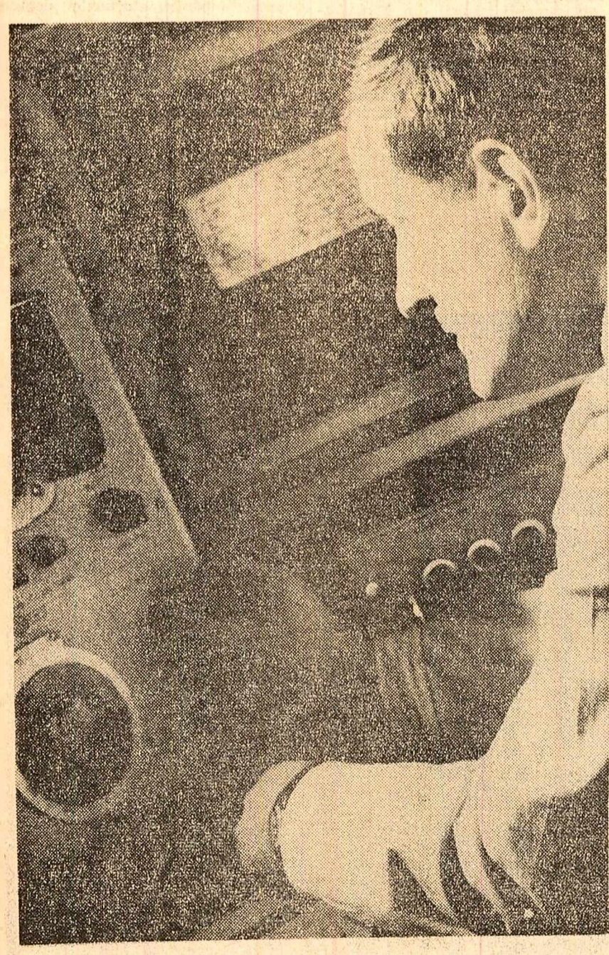
La Observatorul astronomic din Capitală
