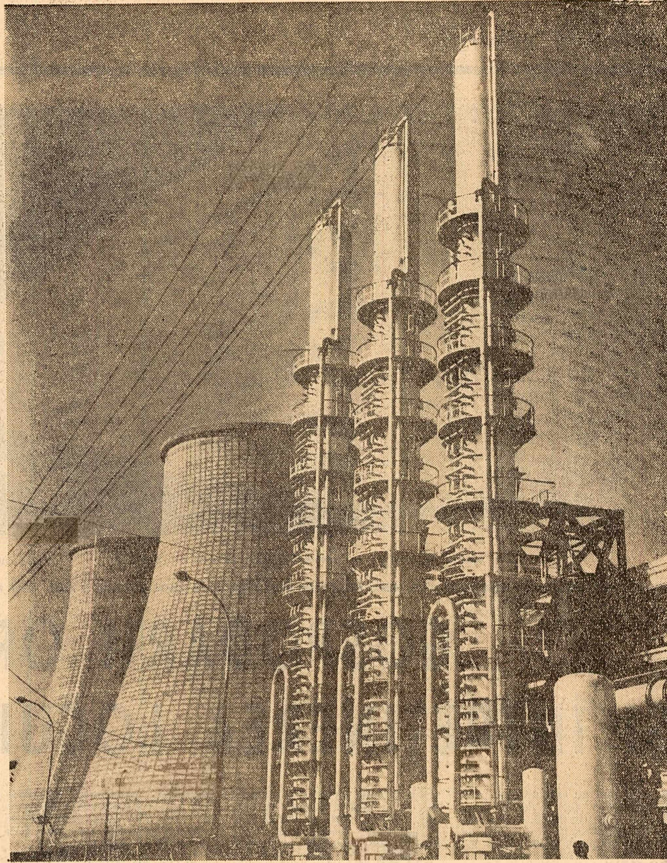
Combinatul de îngrășăminte chimice din Tg. Mureș. Coloanele de absorbție ale fabricii de acid azotic și turnurile de răcire. Foto: A. Cartoian
