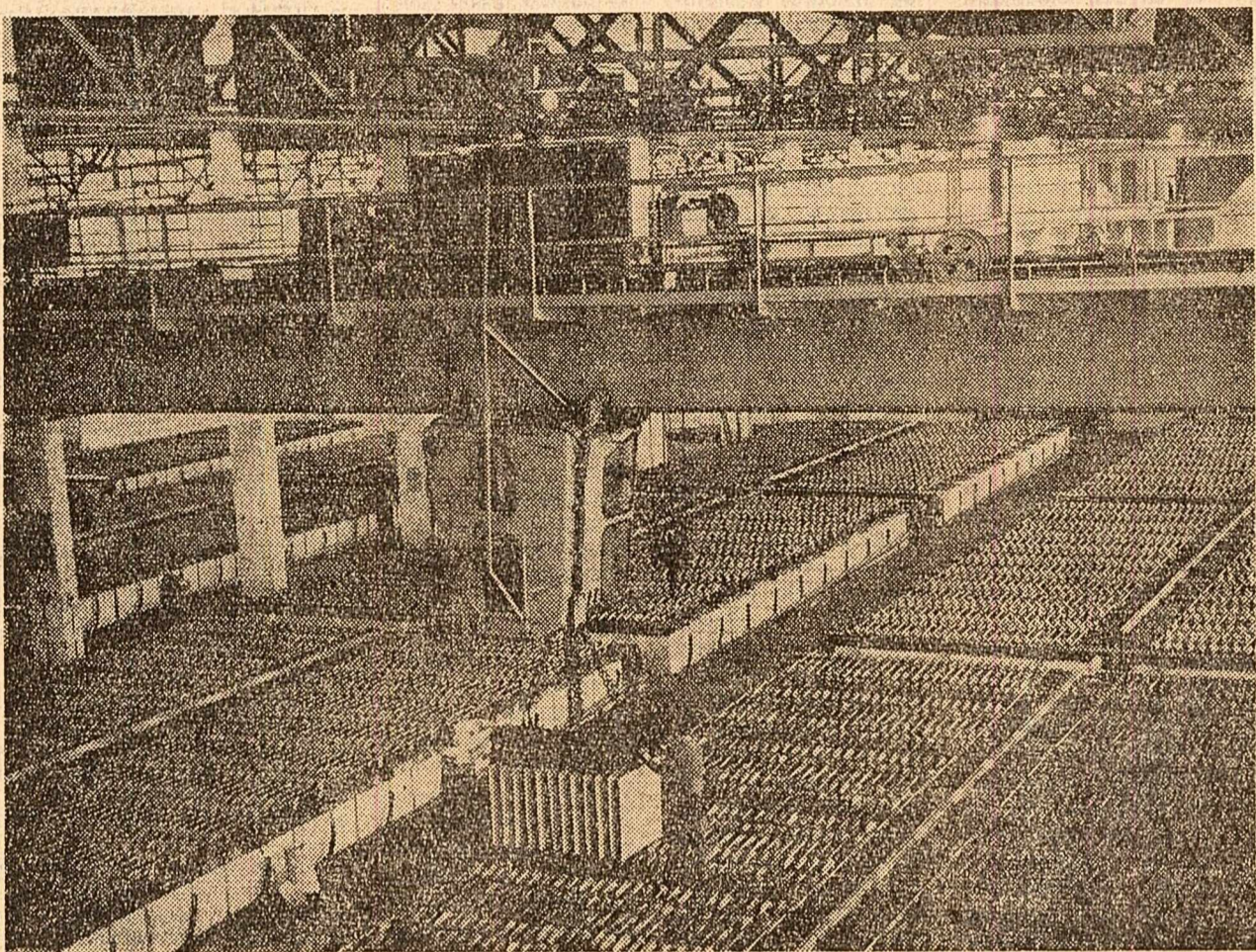
Secția electroliță din cadrul Combinatului chimico-metalurgic „Gheorghe Gheorghiu-Dej” — Baia Mare Foto: A. Carțoian
