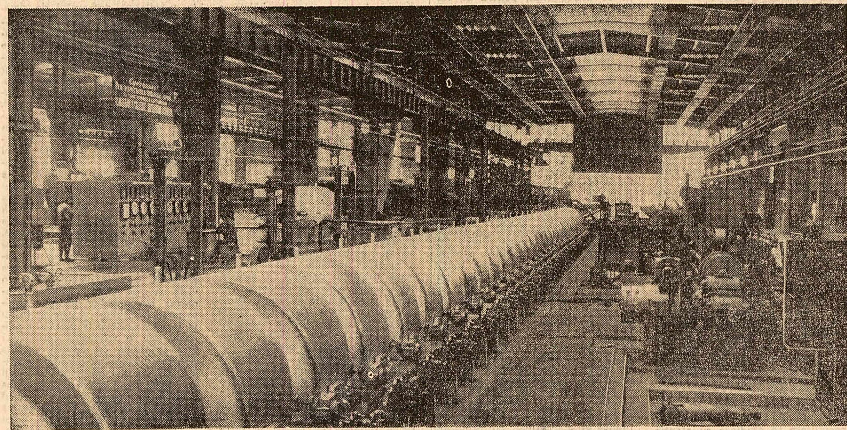
Cuprul tunel și linia de sudură automată a țevilor de la Uzina metalurgică din Iași
