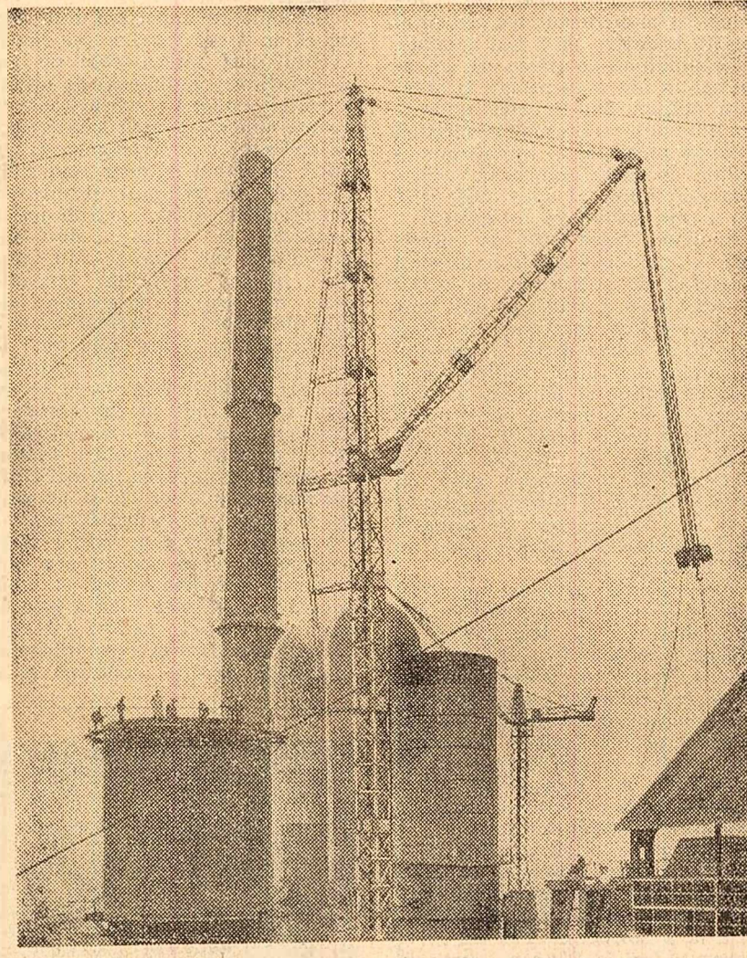
Se lucrează intens la construcția noului furnal de 1000 mc de la Combinatul siderurgic Hunedoara
