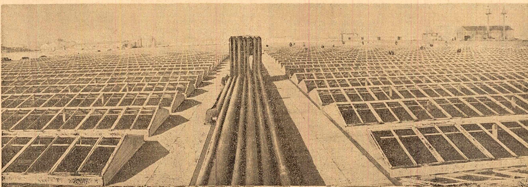
Cîmpul de răsadnile, în suprafață de 3 ha, aparținînd G.A.S. Sabarul-București, este încălzit cu ajutorul apei fierbinți, care circulă prin țevi îngropate în pămînt. Aci se produc mari cantități de legume timpurii, precum și cartofi care vor fi livrați în a doua jumătate a lunii martie. Foto: J. Agerpres
