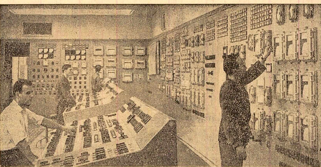
La întreprinderea electrocentrală București a fost dată recent în funcțiune o nouă sală de mașini. Redăm în imagini: sus, sala mașinilor de 50 MW, jos, camera de comandă
