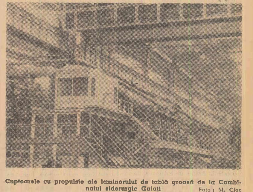
Cuptorul cu propulsie ale laminului de tablă grosă de la Combinatul siderurgic Galați. Foto: M. Cloe
