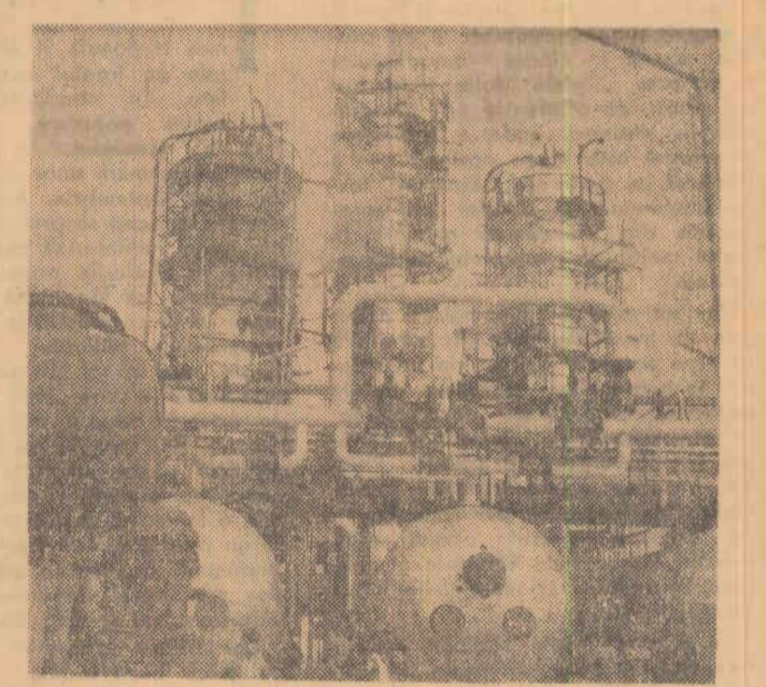
Fabrica de propan-butan a rafinării de la Százhalombatta (R. P. Ungară)
