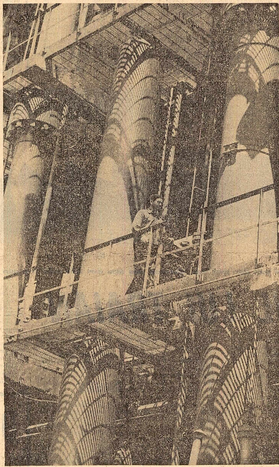
Combinatul chimic Făgăraș. Instalația pentru oxidul și bioxidul de carbon necesar producției de amoniac
