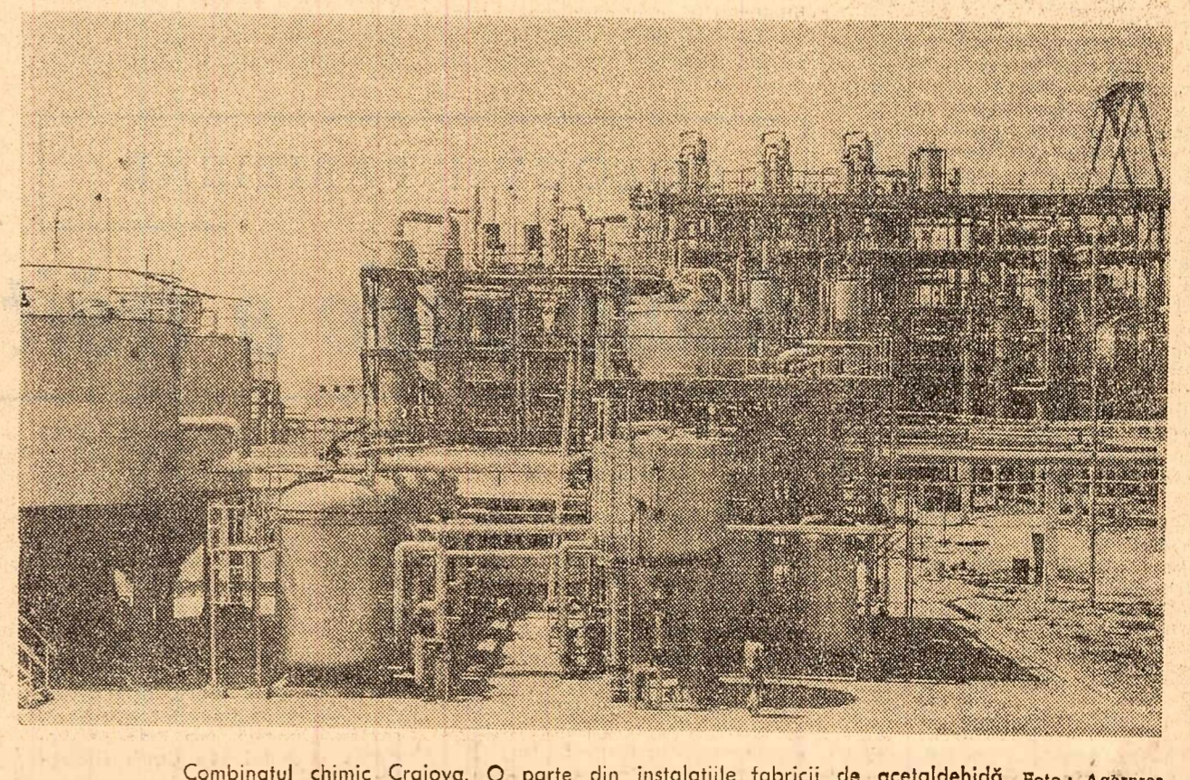
Combinatul chimic Craiova. O parte din instalațiile fabricii de acetaldehidă Foto: Agăpres
