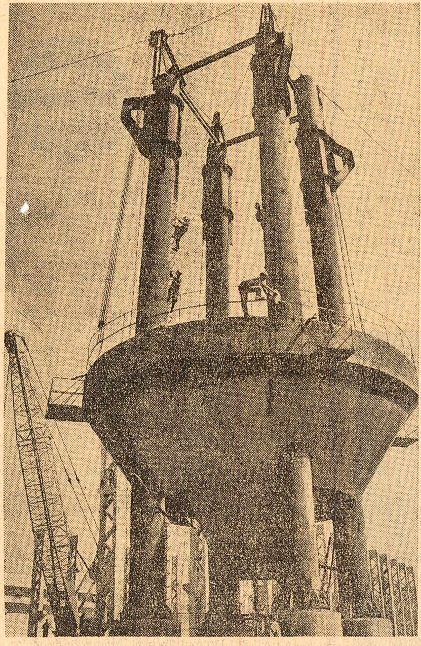
Slatina: Se montează silozul de alumina al halei nr. 3 electroliză Foto: R. Costin
