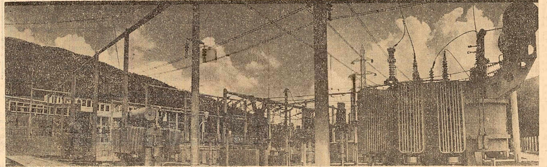
Noua stație de transformare de 110/25 Kv de la Valea Uraș, regiunea Ploiești — una din cele două destinate alimentării cu energie electrică a căii ferate electrice București-Brașov
