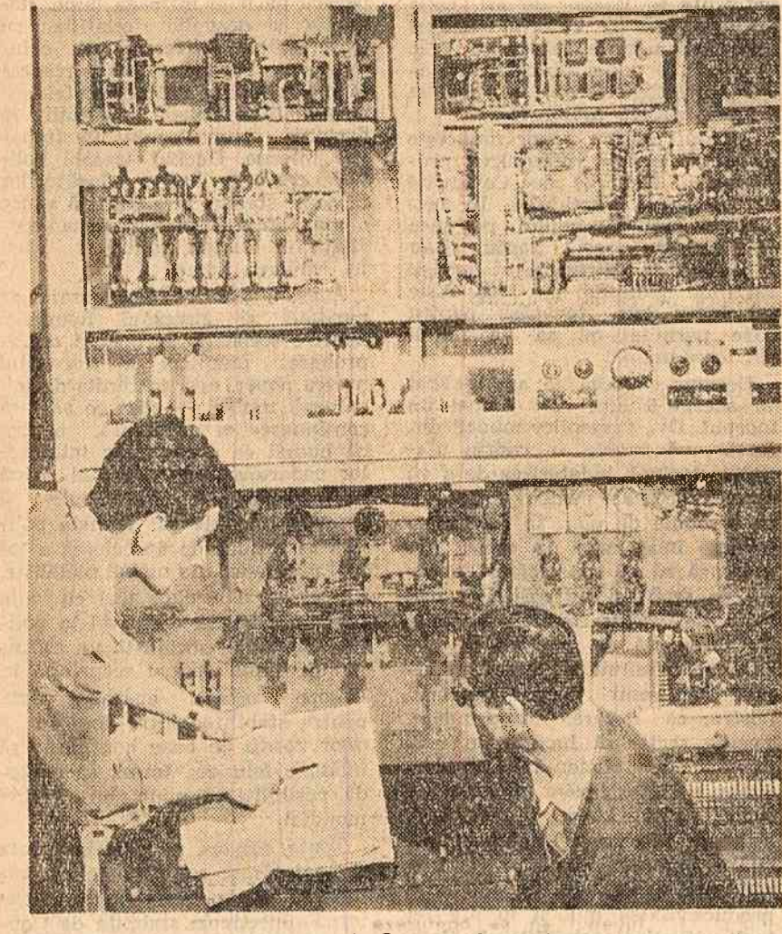
Întreprinderea "Electrotehnica" din Capitală. Se verifică un nou dulap de comandă pentru motoarele Diesel electrice de 400 kW. Foto: Agerpres
