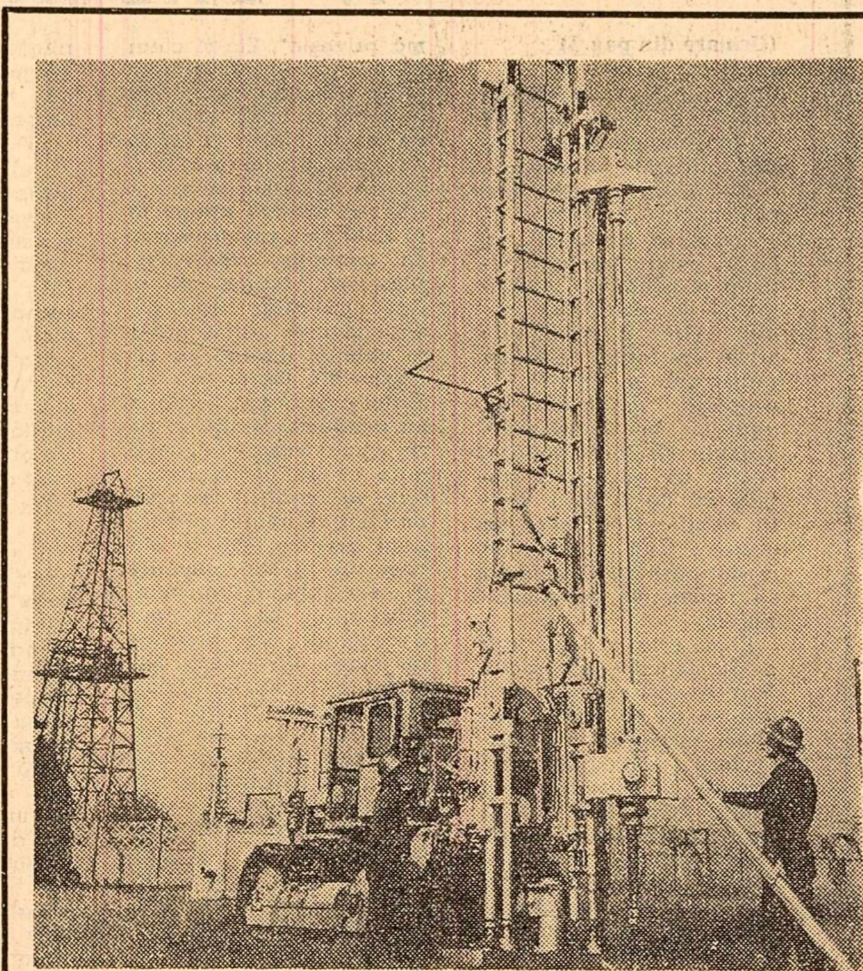
Montată pe tractorul S-650, noua instalație de foraj geologic (în fotografie) poate efectua foraje pînă la adîncimi de 150 m.
