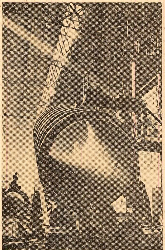
Pentru sporirea productivității muncii și executarea unor lucrări de bună calitate, la uzina „Vulcan” din Capitală s-a construit un dispozitiv pentru sudură automată în T, la recipientii cu diametru mare. În fotografie: cu acest dispozitiv se execută un tronson pentru conducta termocentraliei Borzești.
