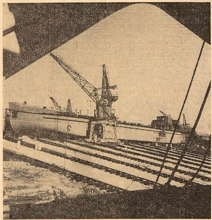
Șantierul naval Oltenija: se finalizează o motonavă de 2.000 tone (Foto Agerpres)
